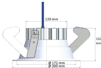
>> Afmetingen armatuur
