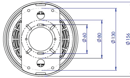
>> Afmetingen armatuur
